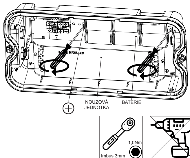
Obrázek. 9 Odpojení a demontáž baterie pomocí křížového šroubováku
