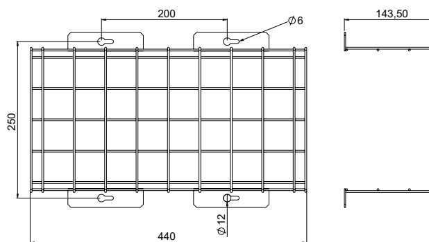
62858 - OCHRANNÝ KOŠ
