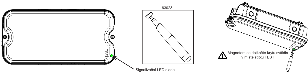
Obrázek 7 Test funkčnosti nouzového systému
