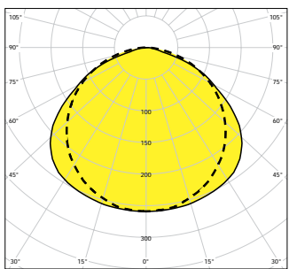
FARGO, 2x58W, IP65 – отражатель белой покраски
