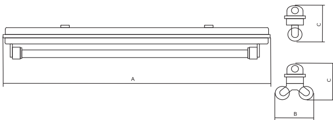
FARGO, 2x58W, IP65 – отражатель белой покраски
